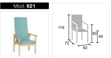
Mod. 621 Sillón respaldo alto. High back chair. Fauteuil grand dossier.
